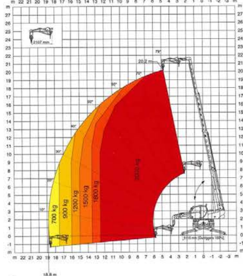
JW 2000 Potence avec treuil 2.000 kg
