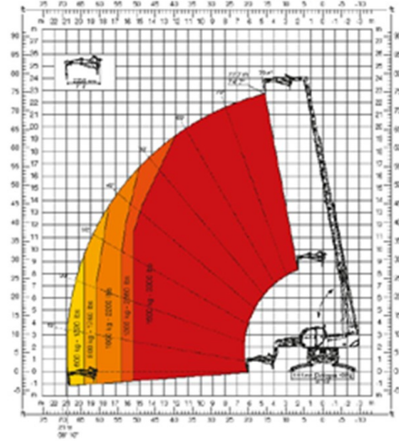
JW 1500 Potence avec treuil 1.500 kg
