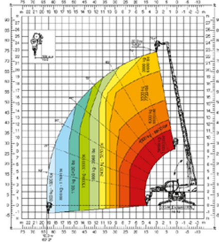
JW 2000 Potence avec treuil 2.000 kg
