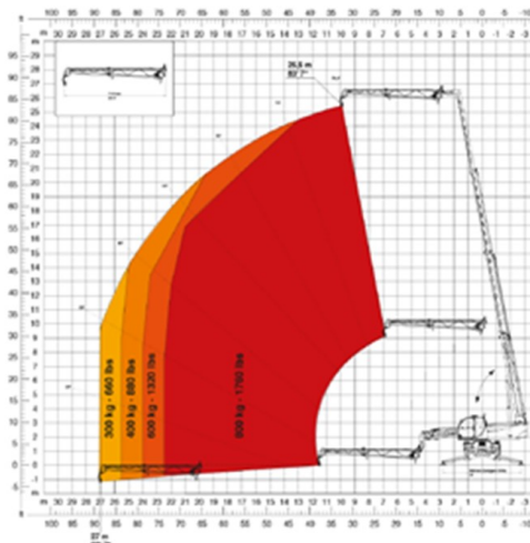
JW 800 potence avec treuil 800
