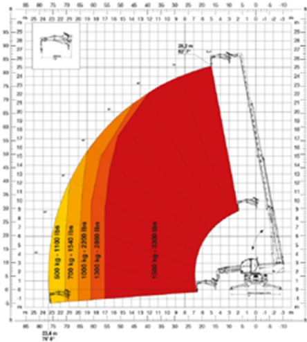
JW 3000 potence avec treuil 3.000
