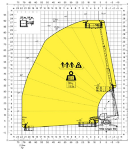
REP 5,2-6,5 W0,3 Nacelle 6,5m 500kg avec treuil 300kg
