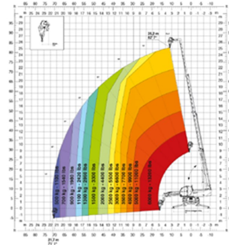
JW 800 potence avec treuil 800
