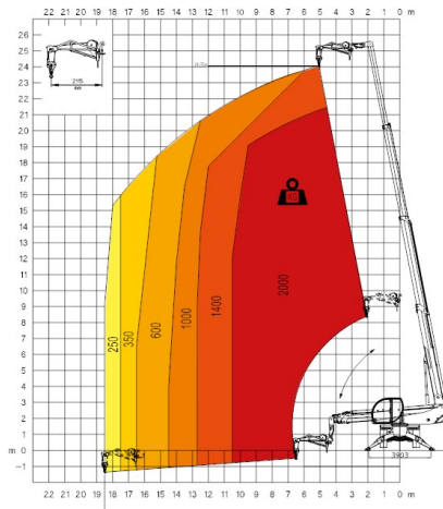
JW 2000 potence avec treuil 2.000
