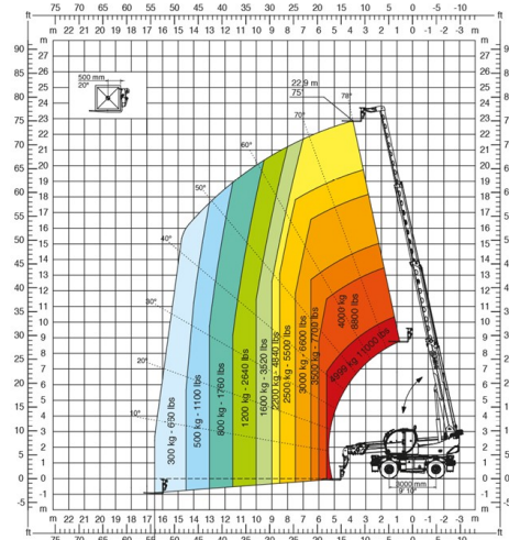
Abaque de charge frontale sur pneus avec fourches
