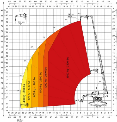
JW 1500 Potence avec treuil 1.500 kg
