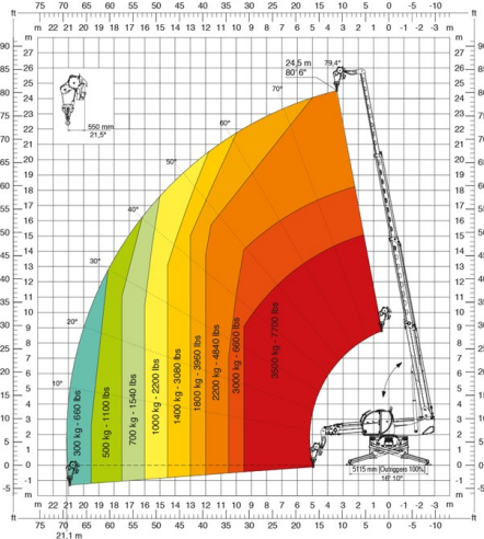
W 3,5 Treuil 3,5 tonnes
