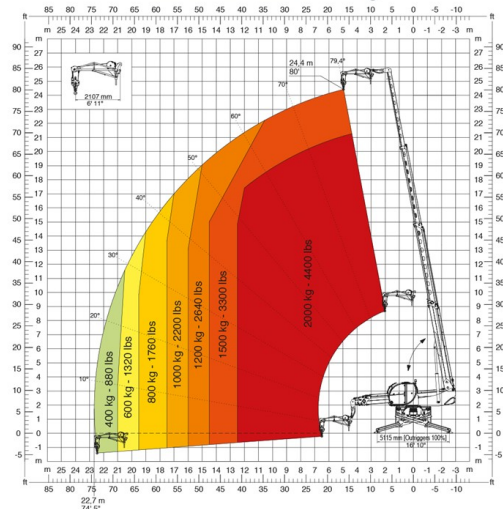
JW 2000 Potence avec treuil 2.000 kg
